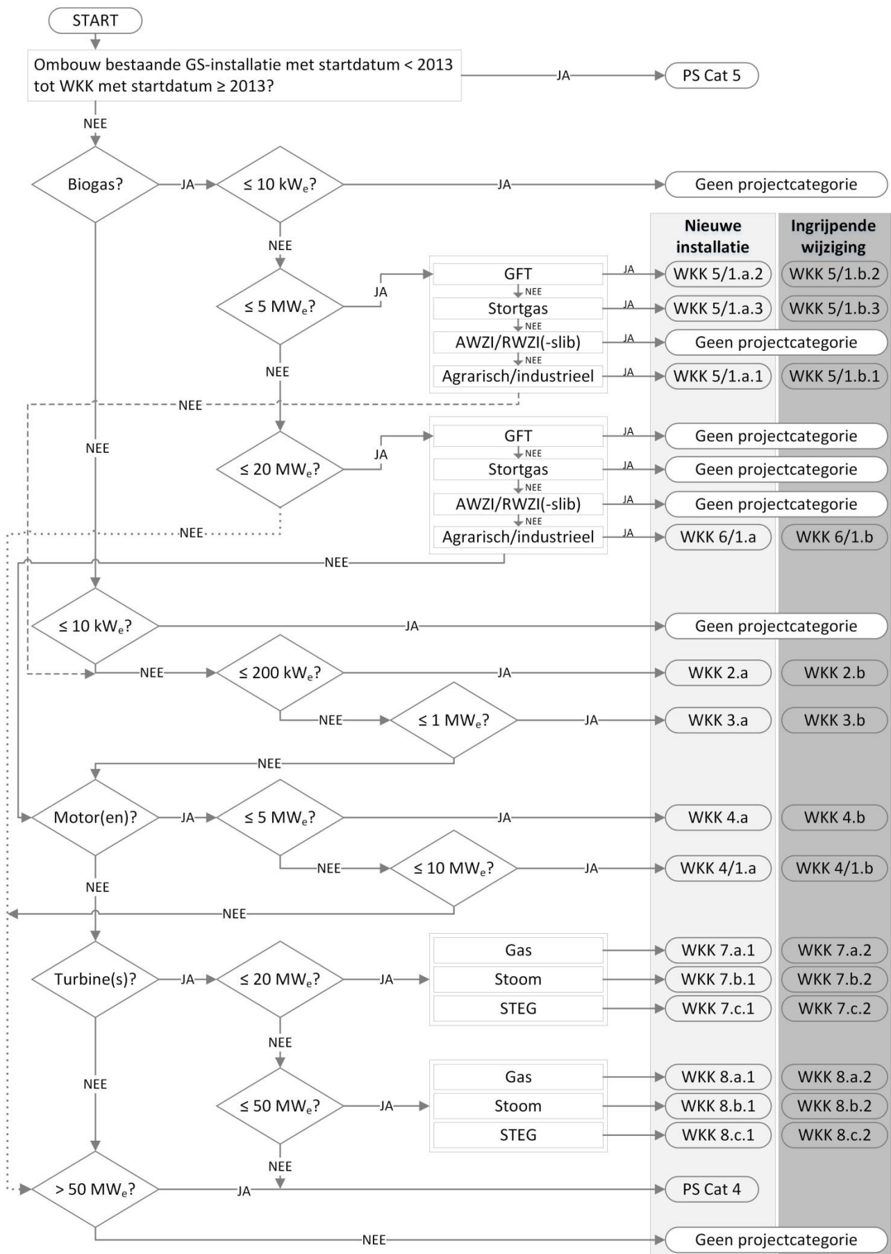
Figuur 2: Stroomschema voor het vaststellen van de WKK-projectcategorie voor projecten met startdatum vanaf 1 januari 2018 (PS: projectspecifiek)
