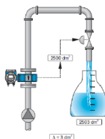
Figuur 20: principe van een volumetrische kalibratie van een debietmeter
