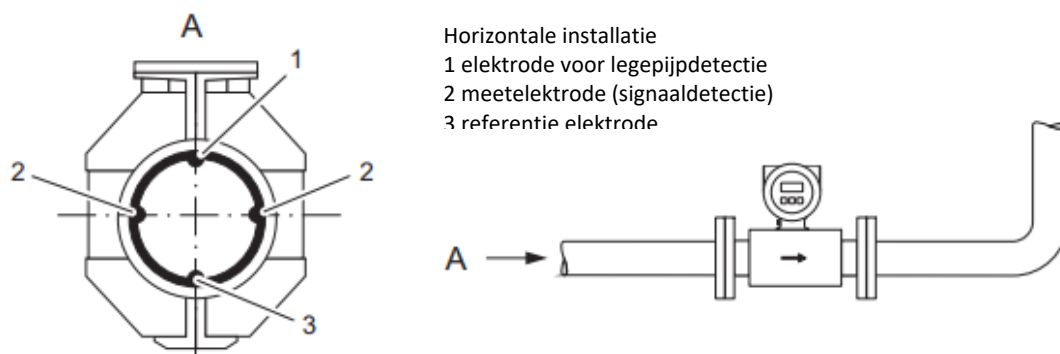
Figuur 11: positie van de elektrodes bij horizontale installatie van een elektromagnetische debietmeter. De meetelektrode (2) moet in de horizontale as liggen om te vermijden dat luchtballen of gesedimenteerde deeltjes het signaal verstoren. De legepijpdetectie (1) moet naar boven gericht zijn (signaalomvormer naar boven gepositioneerd) om de goede werking ervan te garanderen.
