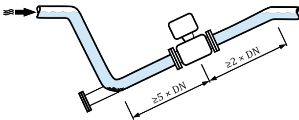
Figuur 9: voorbeeld van een installatie van een elektromagnetische debietmeter met onderhoudspunten [bron: ISO 20456:2017]
