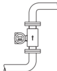
Figuur 10: verticale installatie van een elektromagnetische debietmeter
