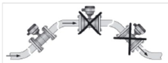
Figuur 15: correcte installatie in gebogen leiding (links); foutieve installatie op hoogste punt (midden) en in gebogen leiding (rechts)
