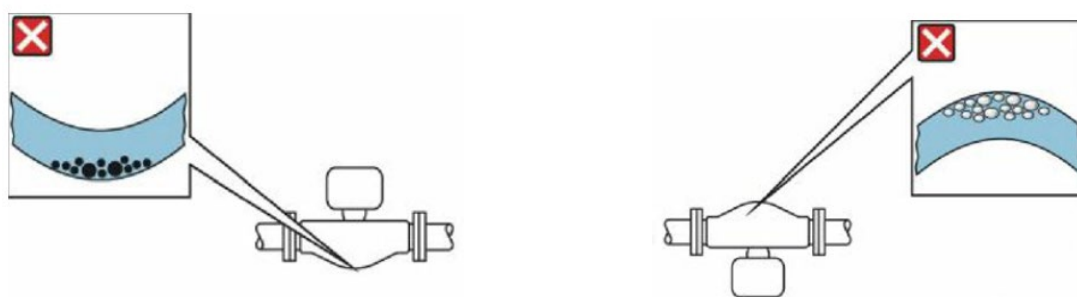
Figuur 12: te vermijden installatie van een coriolismeter bij mogelijkheid tot neerslaan van deeltjes
